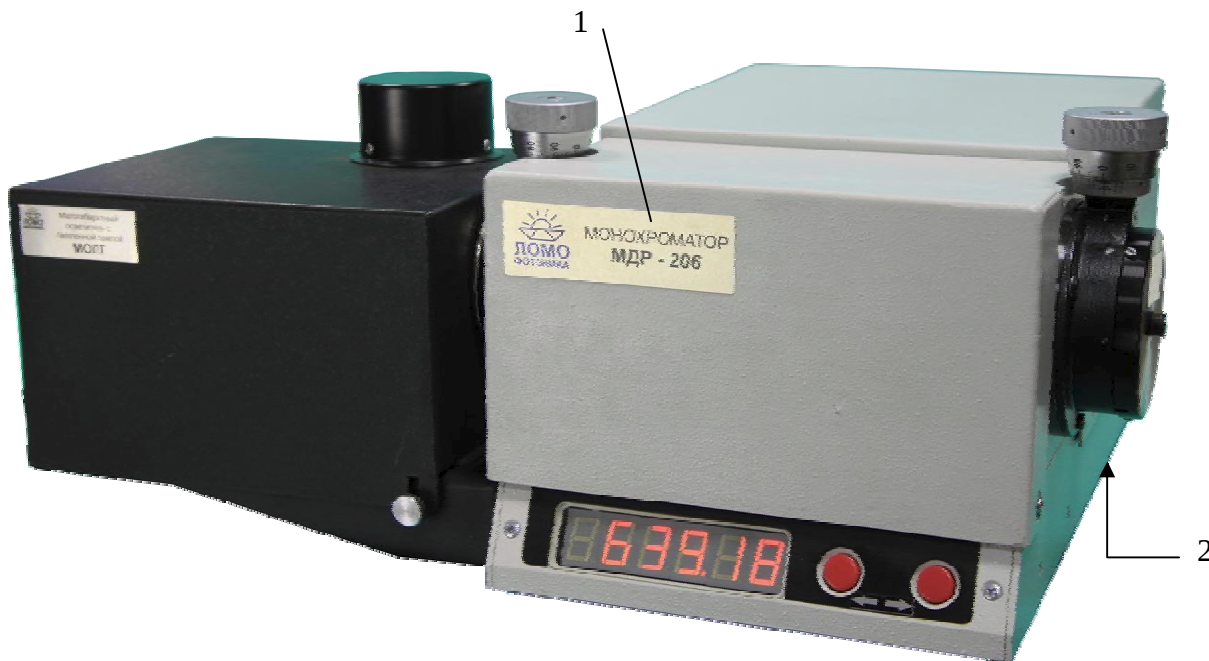
Рисунок 2 - Общий вид, места пломбирования и маркировки монохроматора спектральной установки
